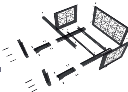
Сборка элементов
