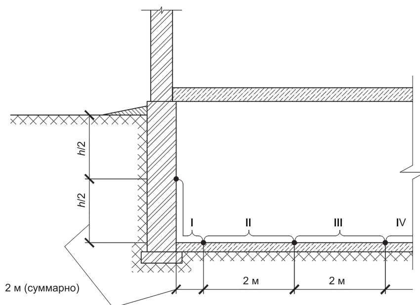
Рисунок Г.1 — Деление на зоны пола по грунту
